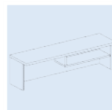
1226 Полка настольная 1200x330x345
